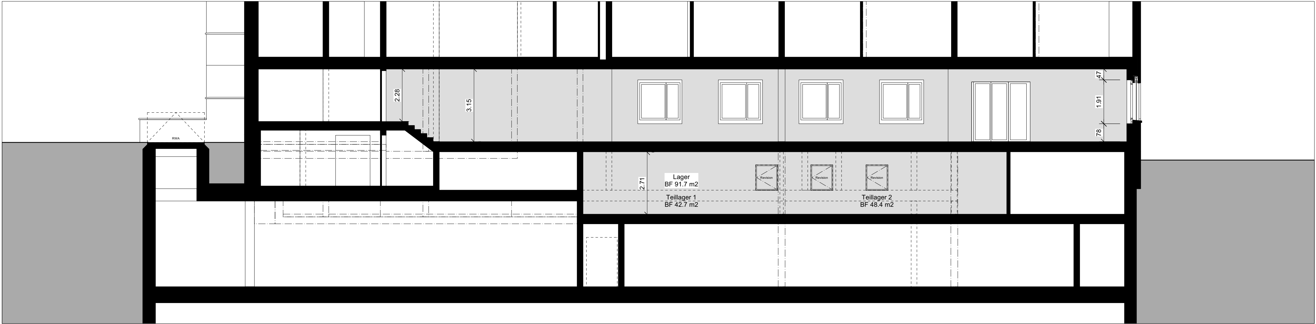
SCHNITT 2E', MST: 1:100
