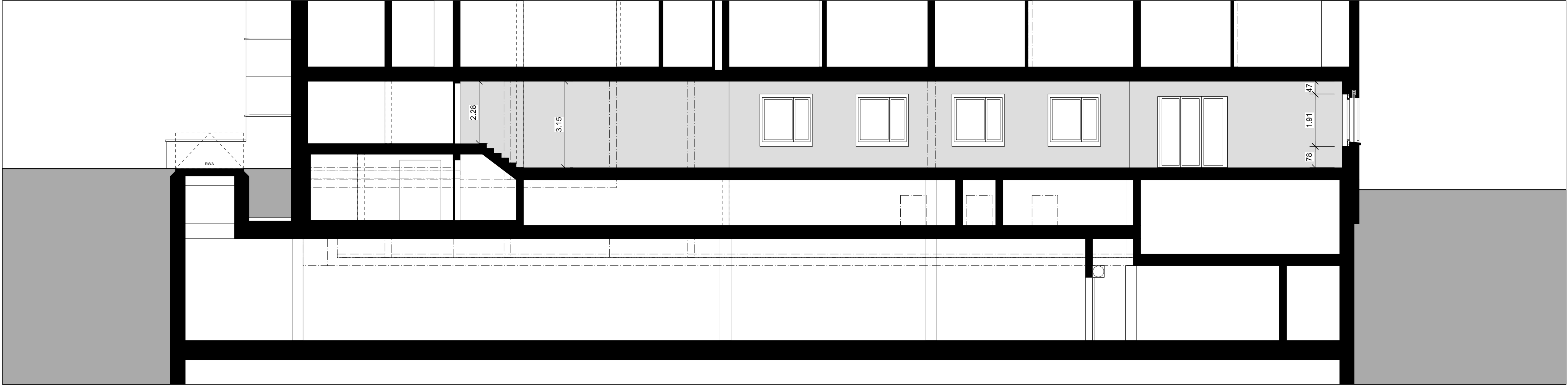
SCHNITT 1E, MST: 1:100
